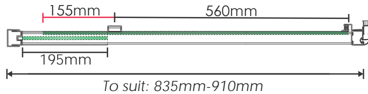
EDEN-T820 (P-Silver) & EDEN T-820B (Black)
